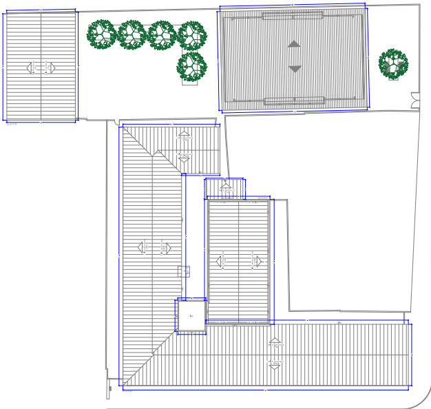
PLANTA BARRA - COBERTURA ESCALA 1:150
